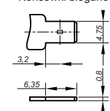
Końcówki biegunowe
