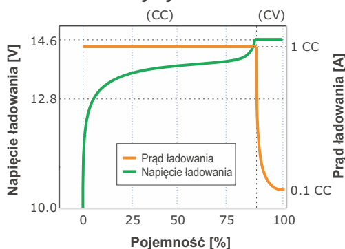
Charakterystyka ładowania
